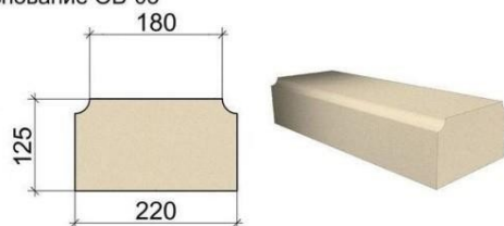
Основание ОВ-03
