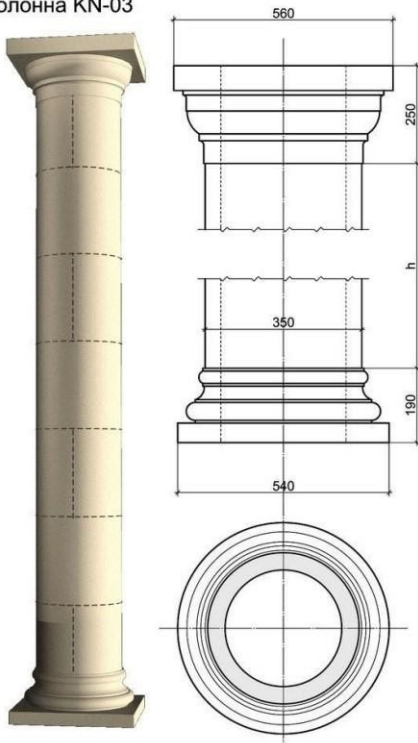
Колонна KN-03
